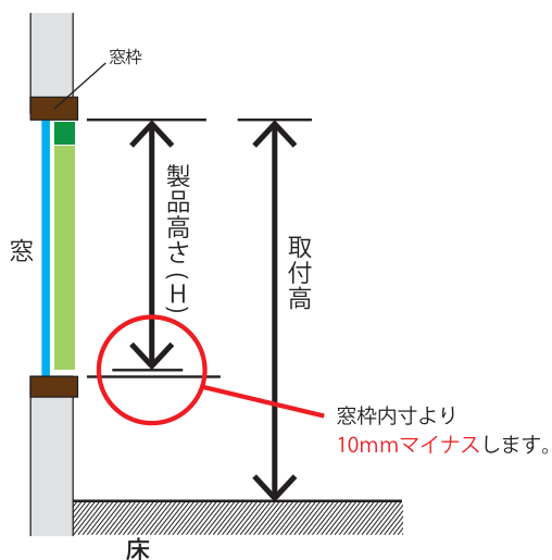
窓枠の内側に取り付ける場合
